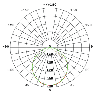
CURVA FOTOMETRICA
